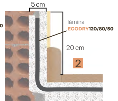
OPCIÓN 2: Retranqueo: Insertar la lámina dentro del muro haciendo un retranqueo.
