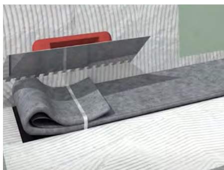
11. Adherir con cemento cola clase C2 S1/S2 sobre encuentros y pendientes la banda ECODRY BANDA termosellada al LINEAL/SUMI LEVEL .
