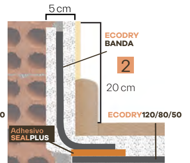
OPCIÓN 2: Retranqueo: Insertar la banda dentro del muro haciendo un retranqueo.
