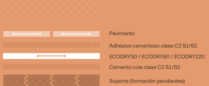
IMPERMEABILIZACIÓN CON LÁMINAS ECODRY50 / ECODRY80 / ECODRY120
